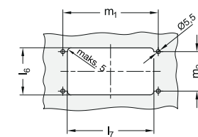
Montaj silüeti
