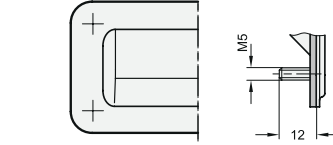
Montaj silüeti
